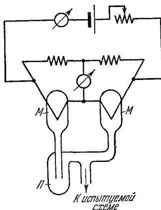
Рис. 2. Схема дифференциального течеискателя.
