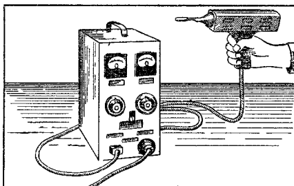
Рис. 1. Галогидный течеискатель.
