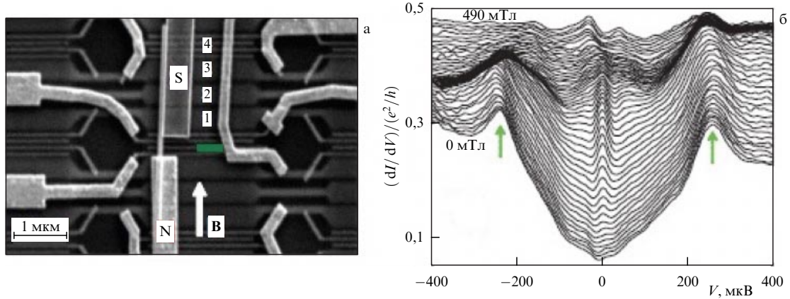
Рис. 11. (а) Изображение InSb-проволоки, которая частично находится в областях нормального, N, и сверхпроводящего, S, контактов в магнитном поле B . 1–4 — затворные электроды. (б) Возникновение пика кондактанса при нулевом напряжении с возрастанием магнитного поля [38].
