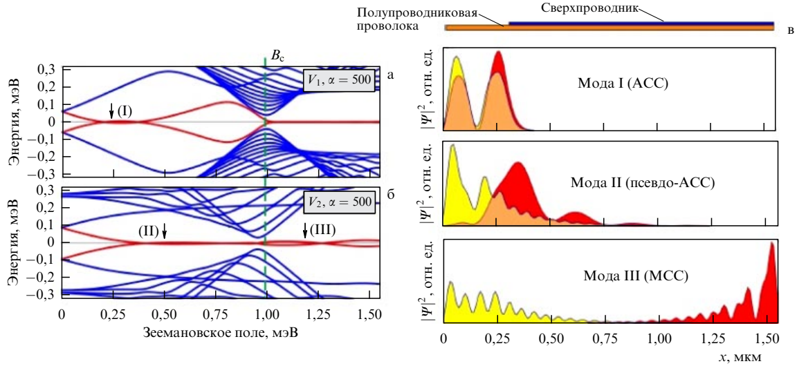
Рис. 12. (В цвете онлайн.) Андреевские и майорановские связанные состояния в системе квантовая точка/сверхпроводящая нанопроволока. Спектры для потенциальных профилей V_1 (а) и V_2 (б). (в) Пространственное распределение плотностей вероятностей майорановских волновых функций для возбуждения с наименьшей энергией (красная кривая на рис. а, б) для различных значений магнитного поля, показанных стрелками на рис. а, б [133].
