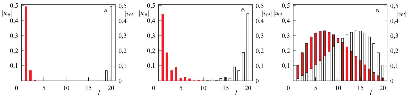
Рис. 5. Пространственные распределения волновых функций майорановских мод при N = 20 для значений параметров, отмеченных на рис. 3 звёздами: (а) |\Delta| = 0,99t , (б) |\Delta| = 0,5t , (в) |\Delta| = 0,1t .
