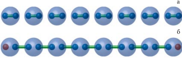
Рис. 1. (В цвете онлайн.) Схематическое изображение слагаемых гамильтониана (4) при (а) t = |A| = 0 , \mu \neq 0 (тривиальный случай) и (б) \mu = 0 , t = |A| (нетривиальный случай). Большие кружки отвечают узлам l , малые — операторам \gamma_{lA} , \gamma_{lB} . Пары операторов, входящих в (4) с ненулевыми коэффициентами, связаны горизонтальными отрезками.
