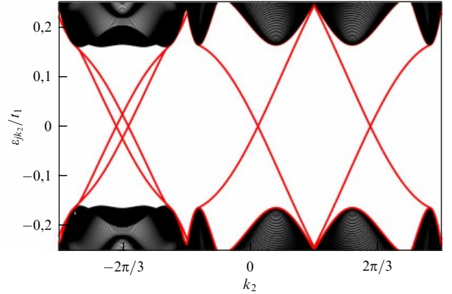
Рис. 31. (В цвете онлайн.) Спектр фермионных возбуждений в фазе сосуществования сверхпроводимости и магнетизма при электронной концентрации n = 1.08 , соответствующей значению топологического инварианта \tilde{N}_3 = -4 , для геометрии цилиндра.
