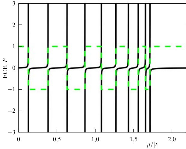
Рис. 7. (В цвете онлайн.) Зависимость величины электрокалорического эффекта (ECE) (сплошная кривая) и индекса фермионной чётности P (штриховая линия по формуле (23)) цепочки Китаева при \Delta/|t| = 0,5 , T/|t| = 10^{-3} и N = 20 .
