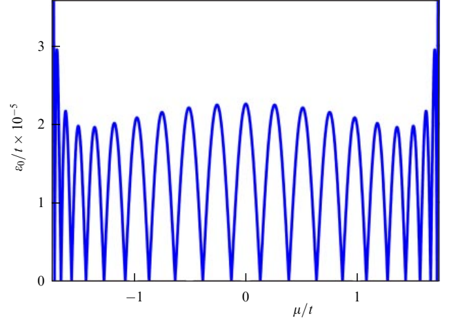
Рис. 4. Зависимость минимальной энергии элементарного возбуждения \varepsilon_0 в цепочке Китаева от химического потенциала \mu при N = 20 и |\Delta|/t = 0,5 (штриховая линия на рис. 3).
