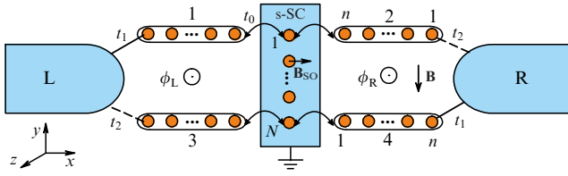
Рис. 16. Кольцо Аарона–Бома, образованное сверхпроводящей нанопроволокой (сверхпроводник s-типа, s-SC), концы которой параллельно связаны с металлическими контактами с помощью подводящих проволок в нормальной фазе [75, 217].
