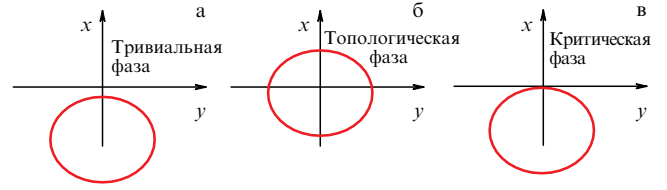
Рис. 2. Схематическое изображение набега фазы Зака–Берри в разных ситуациях: (а) \nu = 0 отвечает тривиальной фазе цепочки Китаева, (б) \nu = 1 — топологической фазе, (в) \nu не определено и отвечает точке топологического квантового фазового перехода.
