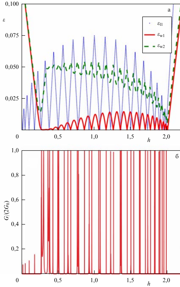
Рис. 17. (В цвете онлайн.) Зависимость (а) энергий одноэлектронных возбуждений проволок рукавов, \varepsilon_{11} , и мостика, \varepsilon_{w1, w2} , и (б) контактанса кольца от энергии магнитного поля, приложенного в плоскости устройства. Параметры: U = V = 0 , \Phi = 0 .
