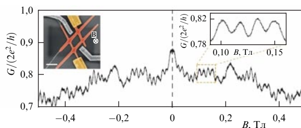
Рис. 15. (В цвете онлайн.) Осцилляции Ааронова–Бомы в кондактансе кольца, изготовленного из проволок InSb (показаны оранжевым цветом на вставке в левой части рисунка) [122].
