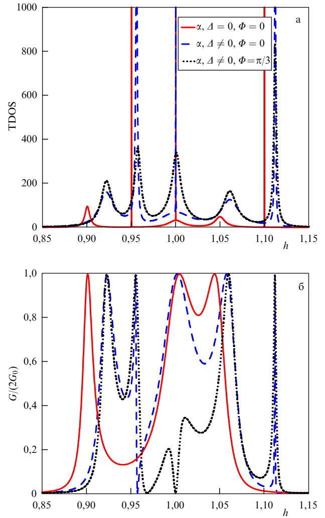
Рис. 18. (В цвете онлайн.) Зависимости плотности состояний (а) и контактанса (б) структуры из шести квантовых точек от энергии магнитного поля при t = 0,1 .
