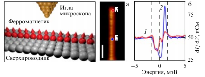
Рис. 27. (В цвете онлайн.) (а) Схема эксперимента по методу сканирующей туннельной спектроскопии со спиновой цепочкой для наблюдения майорановских мод. (б) Зависимость кондактанса от энергии для различных положений иглы микроскопа (1 и 2). Пик при нулевой энергии для зависимости 1 связывается с майорановской модой. Вертикальные штриховые линии, пересекающие ось абсцисс при ненулевых значениях энергии, определяют величину сверхпроводящей щели на свинцовой подложке [233].
