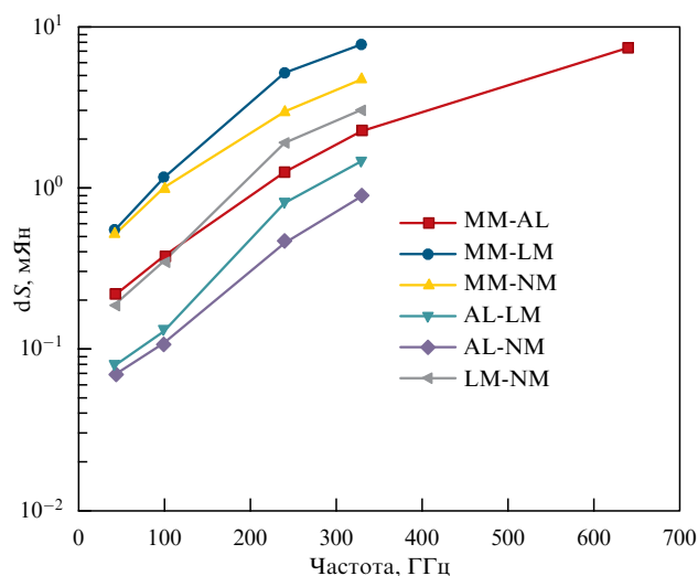
Рис. 1. Сравнительная чувствительность \delta S (ср. кв. отклонение) для некоторых интерферометров космос–Земля с обсерваторией Миллиметрон на частотах 43, 100, 240, 330 и 640 ГГц, \Delta\nu = 4 ГГц; сокращения ММ — Миллиметрон, АЛ — ALMA, LM — LMT (Large Millimeter Telescope), NM — NOEMA (NOthern Extended Millimeter Array).
