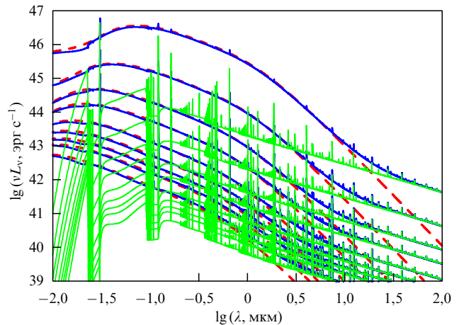
Рис. 14. (В цвете онлайн.) Суммарный спектр OBG: спектр (показан синими линиями), исходящий из аккреционного диска растущей чёрной дыры — красные штриховые линии, и из ионизованного окружающего газа галактики — показан зелёными линиями. Спектр приведён в системе, связанной с чёрной дырой. Масса чёрной дыры увеличивается во времени от 10^5 M_\odot при z = 16 до 9 \times 10^8 M_\odot при z = 8 ; кривые приведены для масс чёрных дыр красных смещений от z = 16 до z = 8 с интервалом \Delta z = 1 снизу вверх (что соответствует точкам на рис. 12). (График взят из работы [144].)
