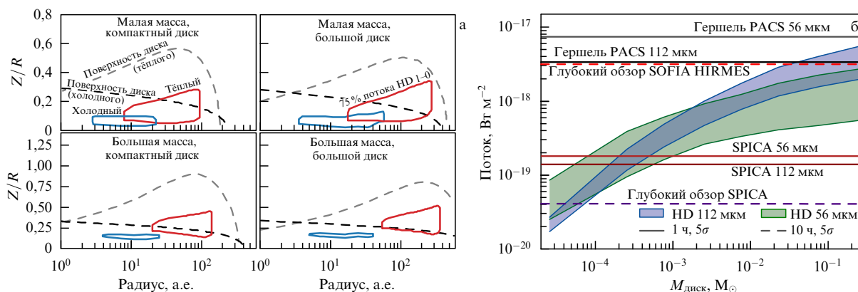
Рис. 19. (а) Модель распределения молекул HD в протопланетных дисках по линии HD\ J = 1 - 0 . Сплошные контуры ограничивают области, включающие 75 % эмиссии в J = 1 - 0 от диска; синие контуры соответствуют тонким (холодным) дискам, красные — толстым (тёплым); штриховые контуры указывают изоконы равной концентрации газа в диске n_g = 10^6\text{ см}^{-3} . В верхнем/нижнем ряду представлены конфигурации для дисков малой/большой массы, левая/правая колонки различают компактные/протяжённые диски. (Рисунок заимствован из работы [262].) (б) Модельная зависимость потока в линиях HD\ J = 1 - 0 (синяя полоса) и HD\ J = 2 - 1 (зелёная полоса) от массы протопланетного диска, расположенного на расстоянии 140 пк. Линиями разного стиля показаны пределы чувствительности некоторых телескопов в дальнем ИК диапазоне: завершивший наблюдательную программу "Гершель" PACS (Photodetector Array Camera and Spectrometer), действующая стратосферная обсерватория SOFIA HIRMES (High Resolution Mid-infrared Spectrometer) и планируемый внеатмосферный телескоп SPICA (SPace Infra-red telescope for Cosmology and Astrophysics), как указано. Чувствительность КОМ в диапазоне 100–300 мкм при охлаждении до 20 К будет почти на два порядка превосходить чувствительность SPICA. (Рисунок заимствован из работы [261].)
