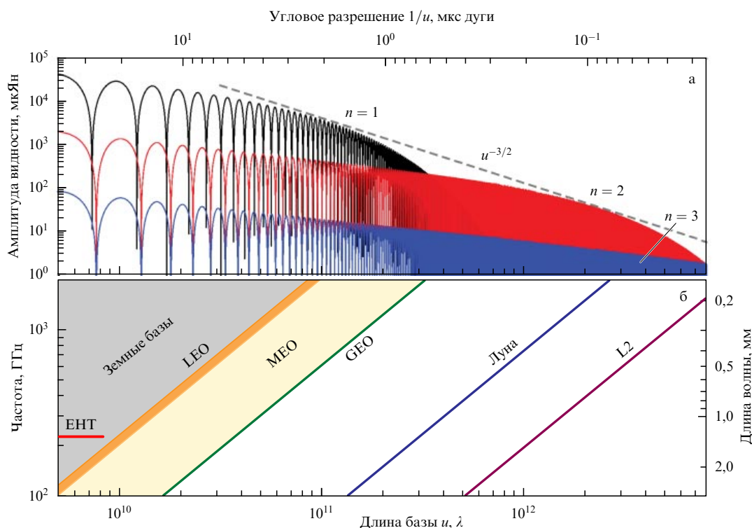
Рис. 17. (В цвете онлайн.) (а) Распределение амплитуды видности в зависимости от длины базы для фотонного кольца с угловым размером \theta = 40 угл. мкс для спектрального потока, сравнимого с потоком от М87. Чёрная, красная и синяя линии соответствуют n = 1 , n = 2 , n = 3 . (б) Приведены базы с размером Земли (соответствуют проекту ЕНТ), с размером близкой (LEO), средней (MEO) околоземной и геостационарной (GEO) орбит, окололунной орбиты (Moon) и точке L2, слева направо. С увеличением размера базы амплитуда видности уменьшается как u^{-3/2} . (График взят из работы [155].)
