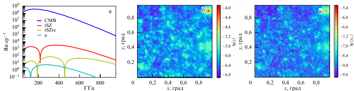
Рис. 4. (В цвете онлайн.) (а) Спектр РИ (синий), спектр y -искажений (красный), первая релятивистская поправка к y -искажениям (жёлтый) и \mu -искажения (голубой). (б) Численная модель карты 1^\circ \times 1^\circ ( 100 \times 100 пикселей) амплитуды y -искажений. (в) Та же карта для первой релятивистской поправки к y -искажениям. Результаты численного моделирования для этих карт были любезно предоставлены Klaus Doulag.
