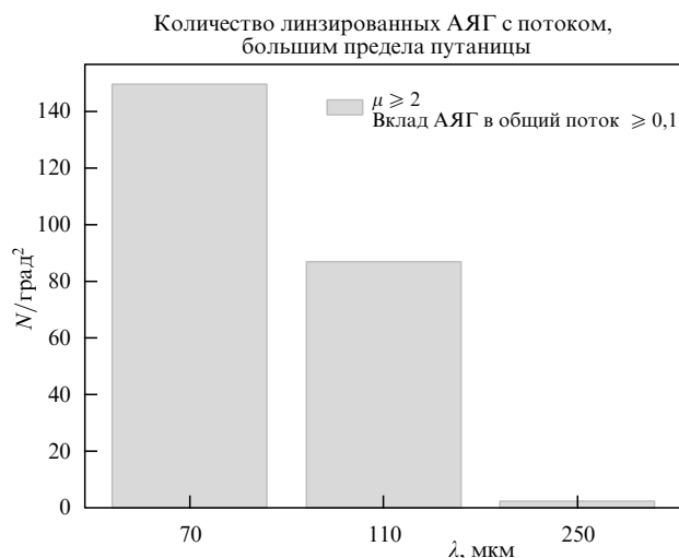
Рис. 8. Количество линзированных АЯГ с коэффициентами усиления \mu \geq 2 в квадратном градусе с потоками, превышающими предел "эффекта путаницы", на длинах волн 70–250 мкм. (Рисунок из работы [62].)
