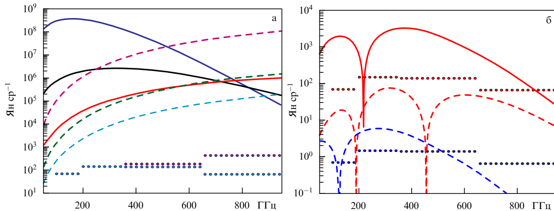
Рис. 5. (В цвете онлайн.) (а) Спектр РИ (синяя линия), вклад от зеркала (чёрная линия), спектр инфракрасного фона (красная линия). Штриховые линии обозначают спектр пыли: фиолетовая — средний спектр по всему небу, зелёная — средний спектр пыли для галактической широты более 30^\circ и голубая линия — спектр пыли для наиболее чистого участка неба. Точками (пунктирными линиями) указана чувствительность Миллиметрона: усреднённая по всему небу — фиолетовый цвет и для наиболее чистого от пыли участка — голубой цвет. (б) \gamma -возмущения — красная сплошная линия, первая релятивистская поправка — красная штриховая линия, \mu -возмущения — синяя штриховая линия. Красная пунктирная линия представляет чувствительность по отношению к \gamma -возмущениям (наблюдательное время 1 час соответствует времени накопления сигнала для каждого отдельного пикселя). Синяя пунктирная линия соответствует времени накопления сигнала для всей карты и представляет чувствительность по отношению к \mu -возмущениям.
