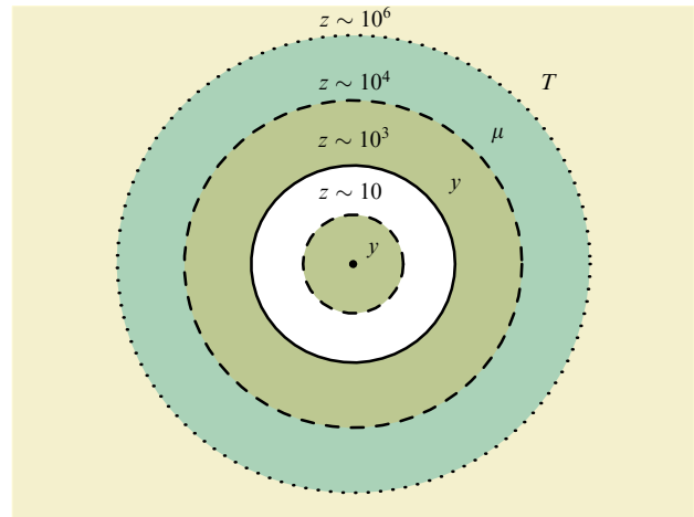
Рис. 3. Этапы эволюции частотного спектра РИ: Т-эра при z > 2 \times 10^6 (сохранение чернотельного спектра), \mu -эра при 5 \times 10^4 < z < 2 \times 10^6 (эра \mu -отклонений) и Y -эра при 1,4 \times 10^3 < z < 5 \times 10^4 и z < 10 (возникновение y -возмущений). Центр рисунка соответствует положению наблюдателя.
