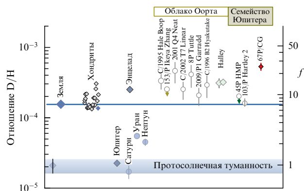
Рис. 22. (В цвете онлайн.) Отношение дейтерия к водороду для планет и малых тел в Солнечной системе. Ромбами показаны данные прямых измерений в различных космических миссиях, кружками — данные, полученные астрономическими методами. Горизонтальными линиями синего и голубого цвета показаны значения соотношения D/H в земном океане и в Солнечной прототуманности. (Рисунок заимствован из работы [346].)
