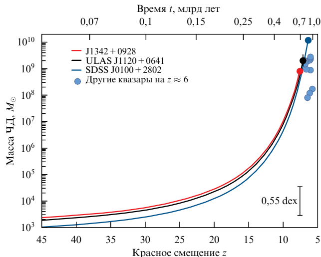
Рис. 12. Рост массы чёрной дыры со светимостью, поддерживаемой на уровне эддингтоновской, и радиационной эффективности 10 % начиная от момента возникновения зародыша ЧД с массами M_{\text{seed}} = 1000 M_\odot — нижняя линия, M_{\text{seed}} \simeq 2000 M_\odot — средняя линия и M_{\text{seed}} = 2500 M_\odot — верхняя линия, при z_0 = 45 ; массы зародышей при z = 45 были выбраны такими, чтобы массы ЧД были равны найденным из наблюдений J1342+0928 ( M_\bullet = 7,8 \times 10^8 M_\odot при z = 7,54 ) [131], ULAS (UKIDSS Large Area Survey, UKIDSS — UKIRT Infrared Deep Sky Survey, UKIRT — United Kingdom Infrared Telescope) J1120+0641 ( M_\bullet = 2,0 \times 10^9 M_\odot при z = 7,09 ) [130], SDSS (Sloan Digital Sky Survey), J0100+2802 ( M_\bullet = 1,2 \times 10^{10} M_\odot при z = 6,33 ) [142].
