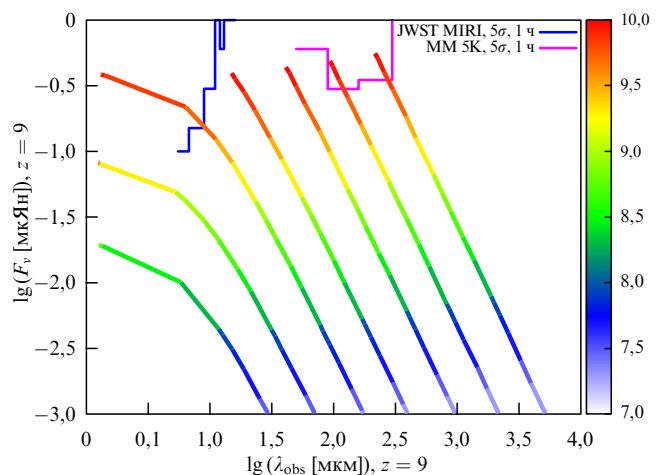
Рис. 15. (В цвете онлайн.) Ожидаемый спектральный поток от растущей чёрной дыры и ионизованного ею газа вблизи частоты излома спектра \nu_k при измерениях с низким спектральным разрешением ( R = 100 ), излучённый на z = 9 , для нескольких значений массы чёрной дыры M_* : 10^5, 10^{5.5}, 10^6, 10^{6.5}, 10^7, 10^{7.5}, 10^8 M_\odot слева направо; цветом вдоль линий показана масса газа в родительской галактике OBG; синяя и фиолетовая линии показывают порог регистрации при времени интегрирования 1 час для телескопов JWST и Миллиметрон. (График из статьи [144].)
