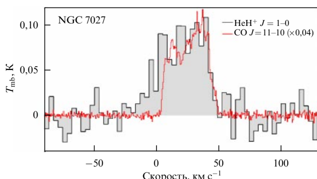
Рис. 20. Спектр вращательного перехода \text{HeH}^+ ( J = 1-0 ), измеренный с помощью upGREAT (German REceiver for Astronomy at Terahertz frequencies с новой версией приёмников) на борту SOFIA в направлении NGC 7027. Для сравнения показана линия CO ( J = 11-10 ), возникающая в плотной молекулярной оболочке вблизи фронта ионизации, откуда, как ожидается, исходит излучение \text{HeH}^+ . (Рисунок заимствован из работы [270].)
