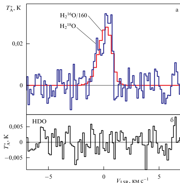
Рис. 23. (В цвете онлайн.) (а) Измеренные при помощи КТ "Гершель"/HIFI спектры перехода 1_{10}-1_{01} для изотопологов H_2^{18}O (линия синего цвета) и H_2^{16}O (линия красного цвета) молекулы воды в комете 45P. (б) Спектр перехода 1_{10}-1_{01} для молекулы HDO. (Рисунок заимствован из работы [348].)
