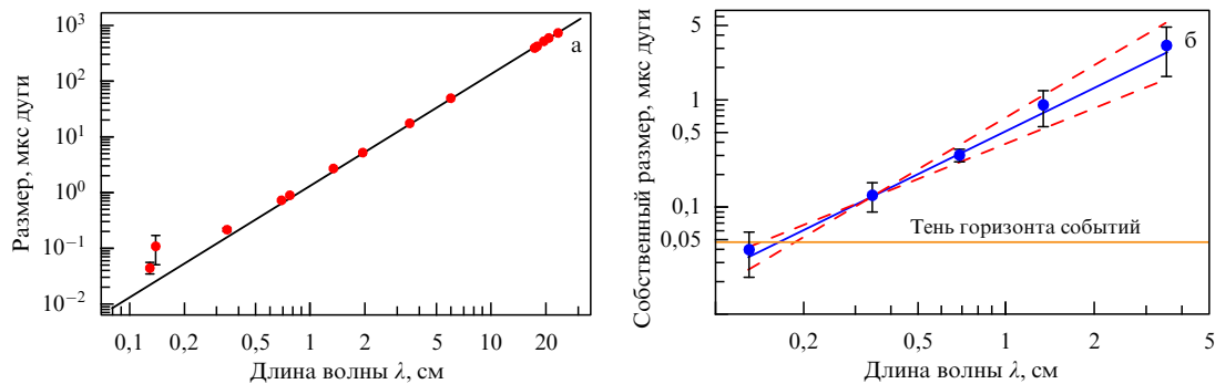
Рис. 16. Эффекты рассеяния при РСДБ наблюдениях источника Sgr A* (см. [157]). (а) Видимый угловой размер источника вдоль большой полуоси в зависимости от длины волны — легко видна зависимость \theta \propto \lambda^2 , обусловленная рассеянием на турбулентных неоднородностях среды. (б) Зависимость видимого углового размера источника после вычитания из наблюдательных точек зависимости \theta \propto \lambda^2 + \text{const} , связанной с вкладом межзвёздной среды — это соответствует близкой окрестности чёрной дыры; горизонтальной линией показан угловой размер тени чёрной дыры. (Из работы [191].)
