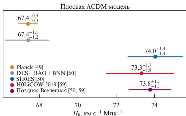
Рис. 7. (В цвете онлайн.) Ограничения на значение постоянной Хаббла для ранней и поздней Вселенной в предположении \Lambda CDM модели. Для ранней Вселенной: оранжевым цветом показан результат обсерватории "Планк" [49] и серым цветом показана комбинация данных, полученных по результатам наблюдений скоплений галактик и слабого линзирования, анализа акустических барионных осцилляций и нуклеосинтеза [60]. Для поздней Вселенной: синим цветом показан результат программы SH0ES [50] и красным цветом — программы H0LiCOW (H0 Lenses in COSMOGRAIL's Wellspring; COSMOGRAIL — COSmological MONitoring of GRAvitational Lenses) [59]. Комбинация двух последних результатов показана малиновым цветом. (Рисунок из работы [59].)
