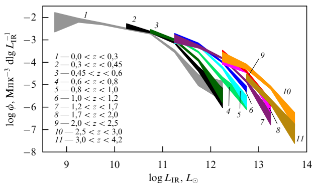
Рис. 11. (В цвете онлайн.) Функция светимости инфракрасных галактик (LIRGs) в интервале красных смещений z = 0-4,2 [124].
