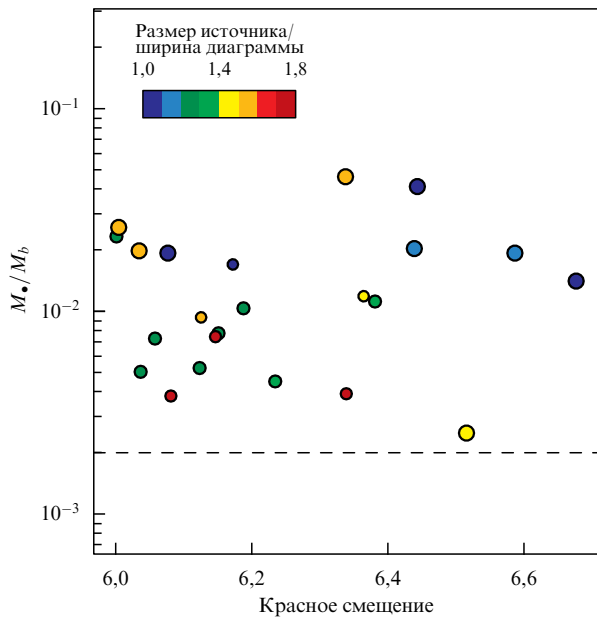
Рис. 13. Отношение массы СМЧД к массе бариев родительской галактики для СМЧД на красных смещениях z \sim 6 ; горизонтальной штриховой линией показано среднее отношение M_*/M_b в современную эпоху z \sim 0 . (График взят из работы [141].)
