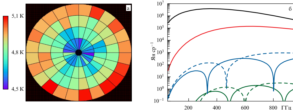
Рис. 6. (В цвете онлайн.) (а) Распределение температуры по поверхности первичного зеркала. 96 панелей имеют различную температуру, которая может увеличиваться от центра к краю на 0,5 К. (б) Вклад от излучения зеркала в общий сигнал. Моменты разложения сигнала \gamma_n B_n : чёрный n = 0 , красный n = 2 , голубой n = 3, 4 , зелёный n = 5, 6 . Штриховыми линиями указаны нечётные моменты ( n = 3, 5 ).
