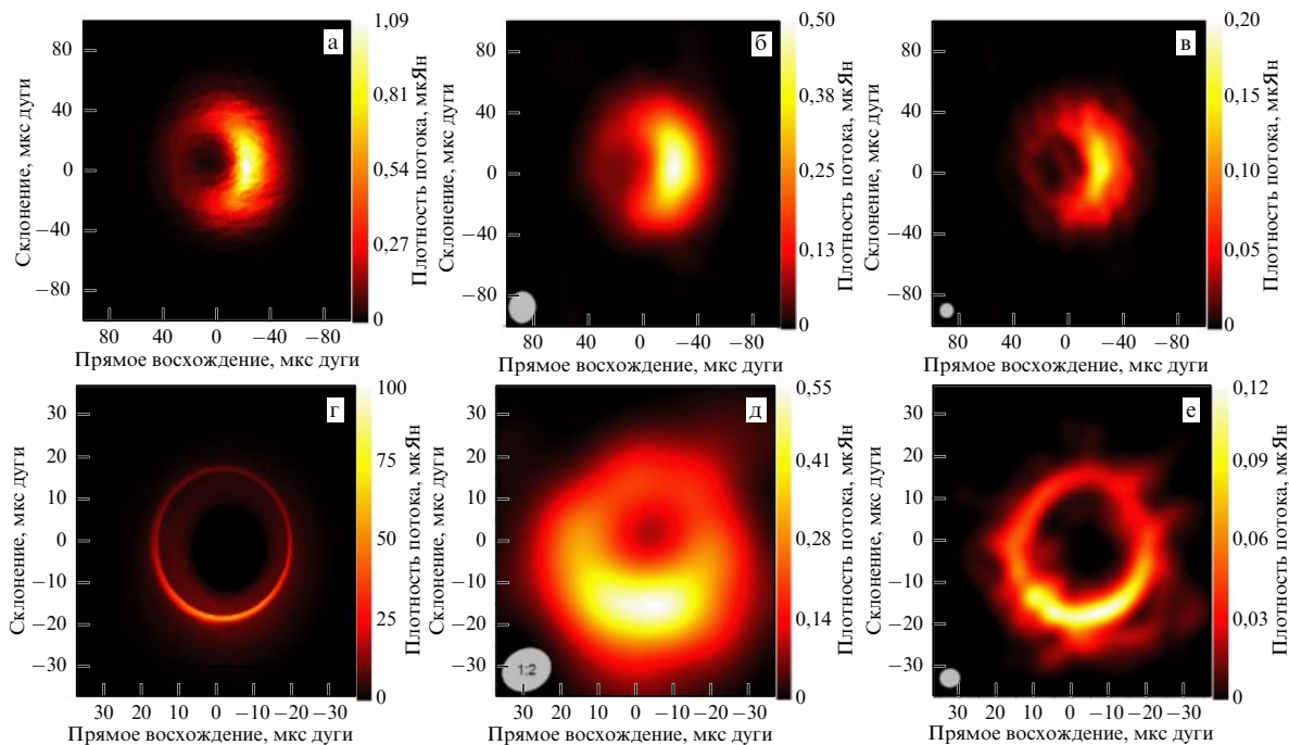
Рис. 18. (В цвете онлайн.) Восстановленные РСДБ изображения источников Sgr A* (а, б, в) и M87 (г, д, е) на частоте 230 ГГц. (а, г) Усреднённые МГД модели ((а) — изображение Sgr A* с учётом рассеяния, (г) — M87* с параметрами, соответствующими наблюдениям ЕНТ 2017 г. [20]). (б, д) Восстановленные РСДБ изображения с использованием наземных телескопов, входящих в ЕНТ. (в, е) Восстановленные РСДБ изображения с использованием наземных телескопов, входящих в ЕНТ, и космического телескопа Миллиметрон на околоземной эллиптической орбите. (Изображения взяты из статьи [23].)
