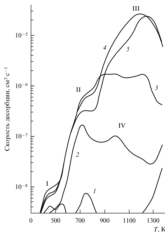
Рис. 5. Кривые температурно-программируемой десорбции (ТПД-пики I–IV) дейтерия из изотропного графита ISO-88, наводороженного при 60 кПа (5 ч) при температурах 473 (I), 673 (2), 773 (3), 973 (4), 1173 K (5) [51].
