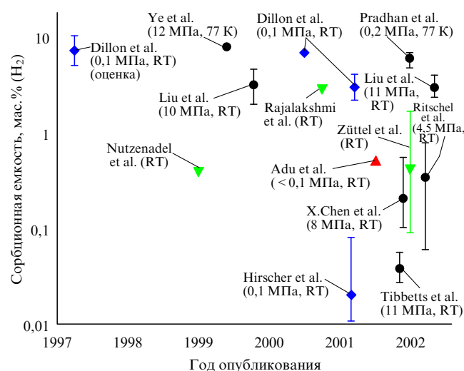
Рис. 4. Данные измерений сорбционной емкости пучков ОСНТ, полученные волуметрическим (●), гравиметрическим (▲), электрохимическим (▼) и ТПД (◆) методами; RT — комнатная температура [8].
