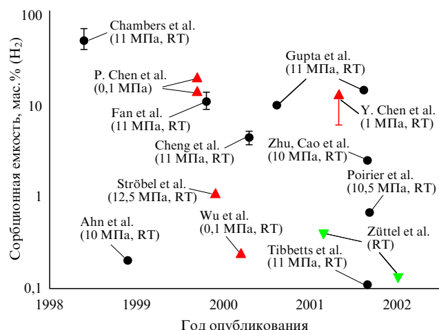
Рис. 3. Данные измерений сорбционной емкости ГНВ и ориентированных УНТ, полученные волуметрическим (●), гравиметрическим (▲) и электрохимическим (▼) методами; RT — комнатная температура [8].
