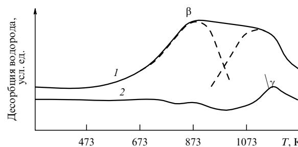
Рис. 6. Кривые температурно-программируемой десорбции — ТПД-пики \beta (II), \gamma (III) водорода из образцов ГНВ, наводороженных при 298 K в течение 24 ч при 11 МПа (1) и 0,1 МПа (2). Штриховые линии — составляющие кривую (1) пики [12].
