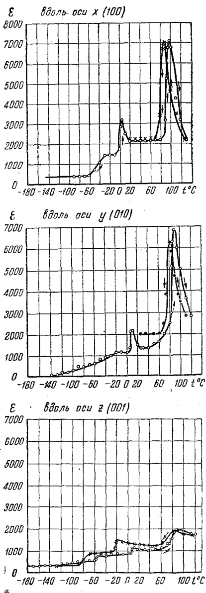
Рис. 13. Температурная зависимость диэлектрической проницаемости монокристалла BaTiO 3 для трёх кристаллографических направлений.
