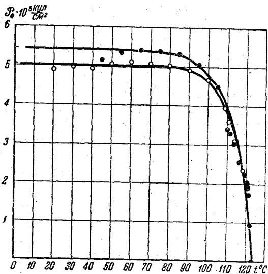
Рис. 9. Температурная зависимость спонтанной поляризации поликристаллических образцов титаната бария.
