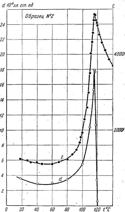
Рис. 18. Температурный ход пьезомодуля и диэлектрической проницаемости, [полученный статическим методом.
