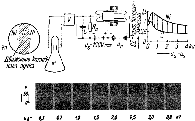
Рис. 5. Схема для получения электрограмм при мощности вторичной эмиссии
