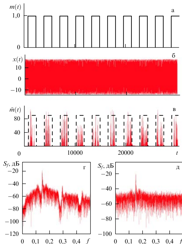
Рис. 11. Иллюстрация численной реализации способа скрытой передачи информации на основе обобщенной хаотической синхронизации в отсутствие шумов и флуктуаций в канале связи ( D = 0 ): (а) информационный сигнал m(t) , представленный простой последовательностью бинарных битов 0/1, (б) сигнал x(t) , производимый передающим генератором для последующей передачи по каналу связи, (в) восстановленный сигнал \hat{m}(t) и детектированный информационный сигнал (штриховая линия). Спектры мощности сигнала в канале связи (г) в отсутствие шума и (д) при шуме интенсивностью D = 10 .
