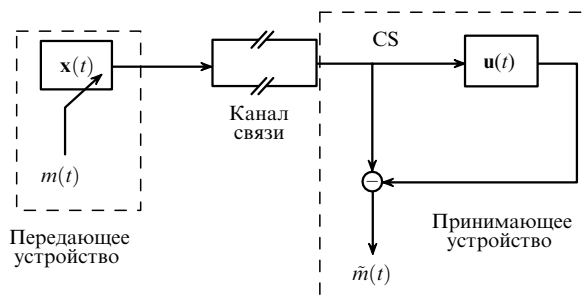
Рис. 5. Схема скрытой передачи информации путём модулирования управляющего параметра передающего генератора информационным сигналом.
