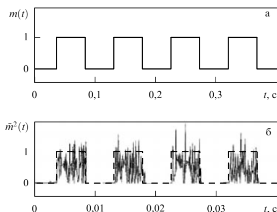
Рис. 15. Иллюстрация экспериментальной реализации схемы передачи информации на основе переключения хаотических режимов: (а) информационный сигнал m(t) , представленный простой последовательностью бинарных битов 0/1, (б) восстановленный в принимающем устройстве сигнал \hat{m}^2(t) (сплошная линия). Штриховой линией представлен детектированный информационный сигнал. (Из работы [189].)
