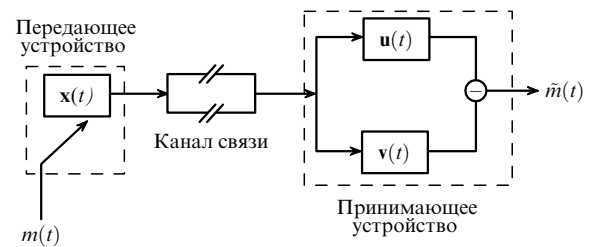
Рис. 10. Схема реализации сверхустойчивого к шумам способа скрытой передачи информации на основе обобщённой хаотической синхронизации.
